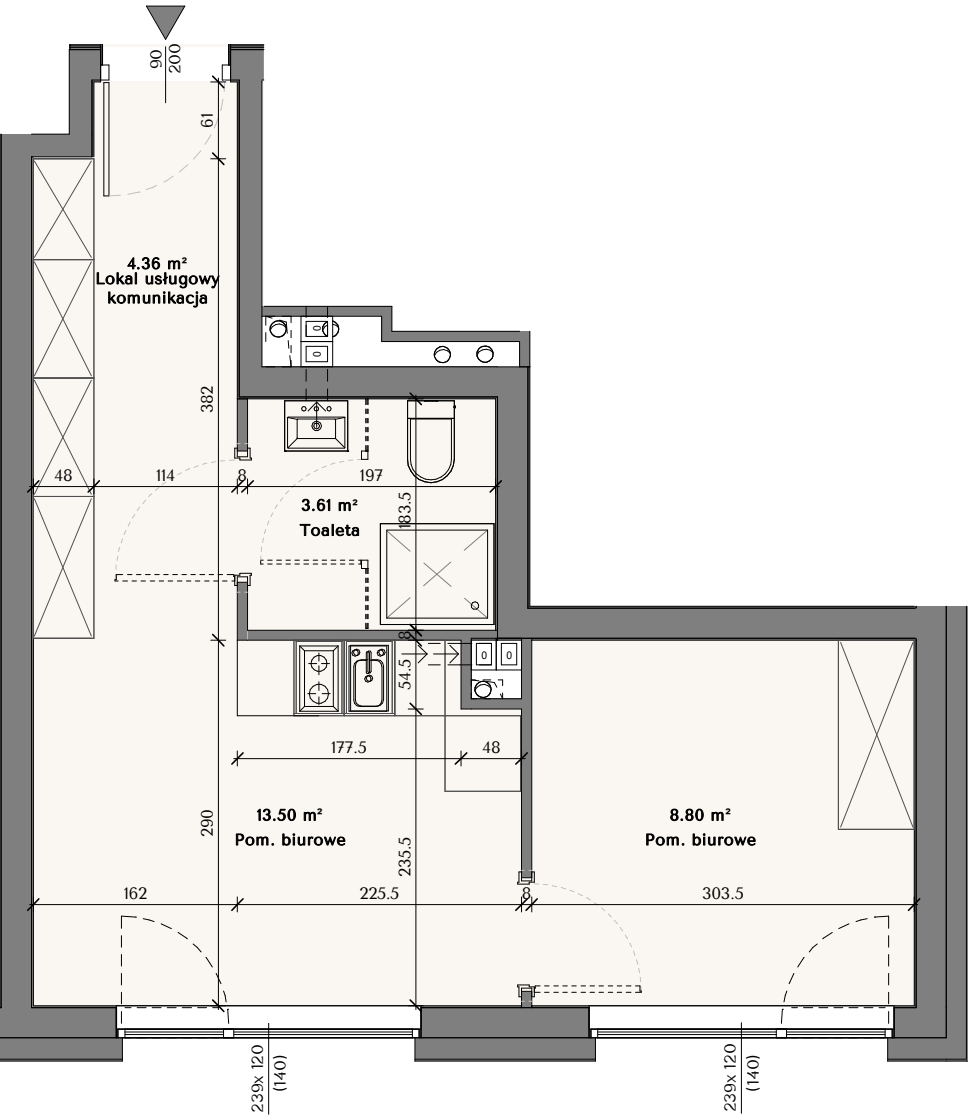
USYTUOWANIE LOKALU NA PARTERZE
